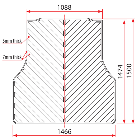
UTM-007 BYD Shark Bed Mat 2024-
